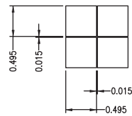
Detail A(S=20:1)
